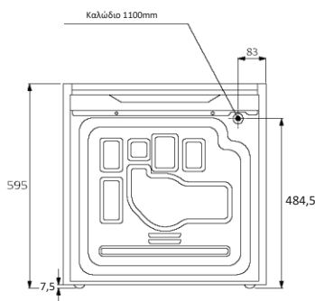
Οπίσθια όψη
