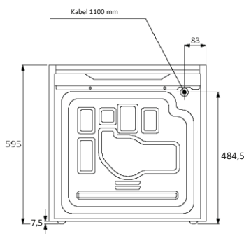
Achteraanzicht
