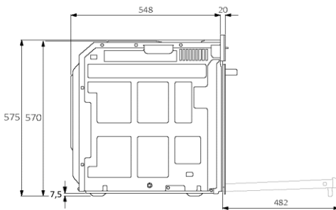
Sivusuunnasta
