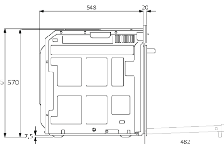
Zijaanzicht
